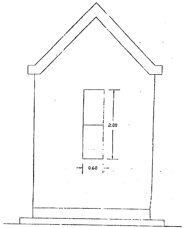
prospetto retro
