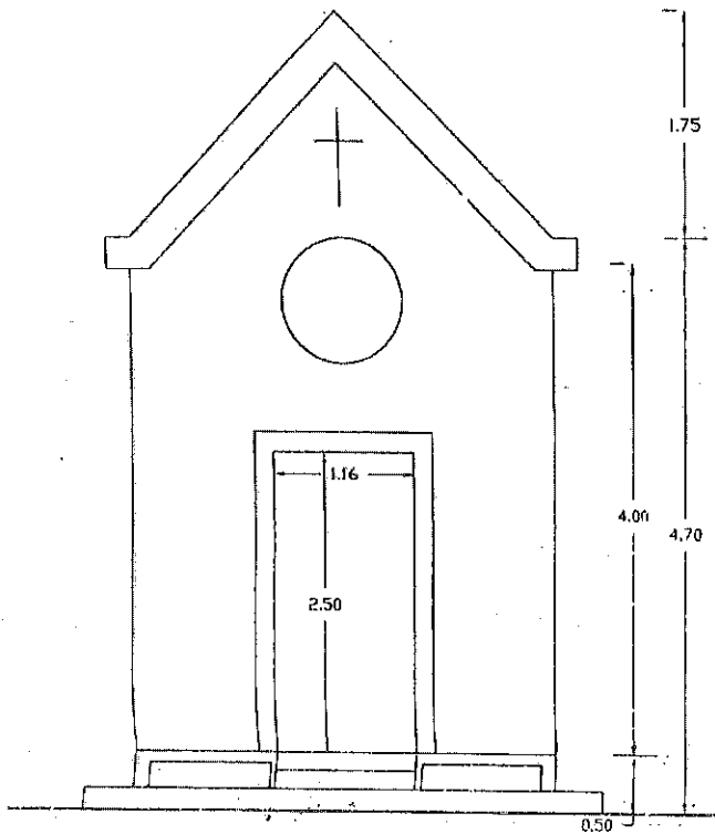
prospetto fronte
