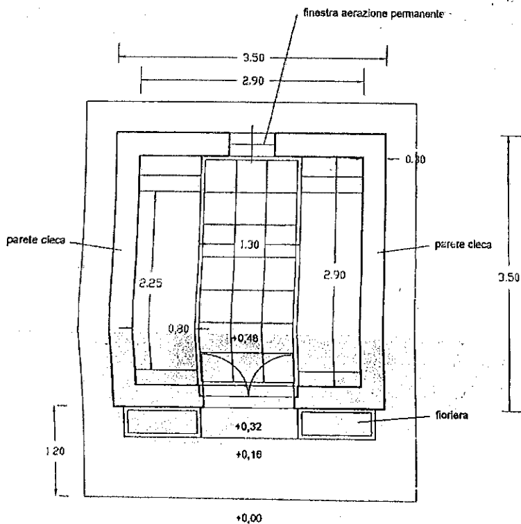
pianta tipo
